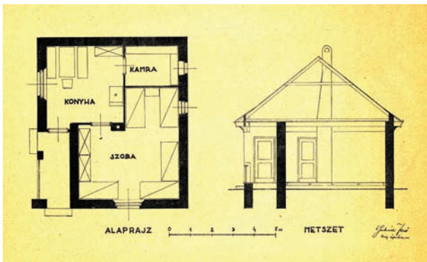
A Komárom vármegyében felépítendő ONCSA-kislakások tervrajza (Forrás: A szociális vármegye, 1941)
